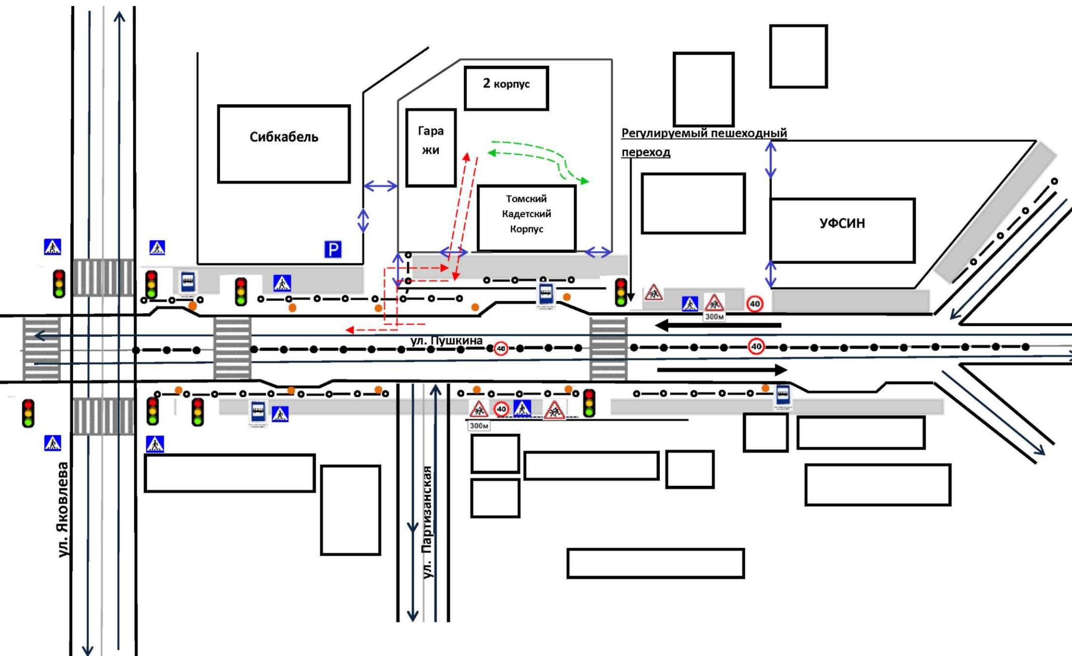
6. План - Схема безопасного расположения детского автобуса у образовательного учреждения.
